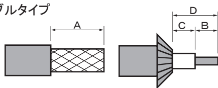
ケーブルカット寸法 同軸ケーブルタイプ
